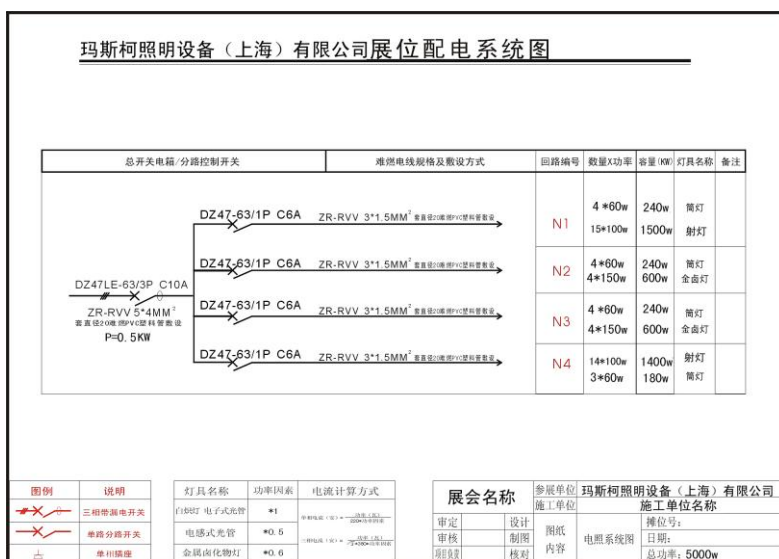
配电系统图 (范本)
